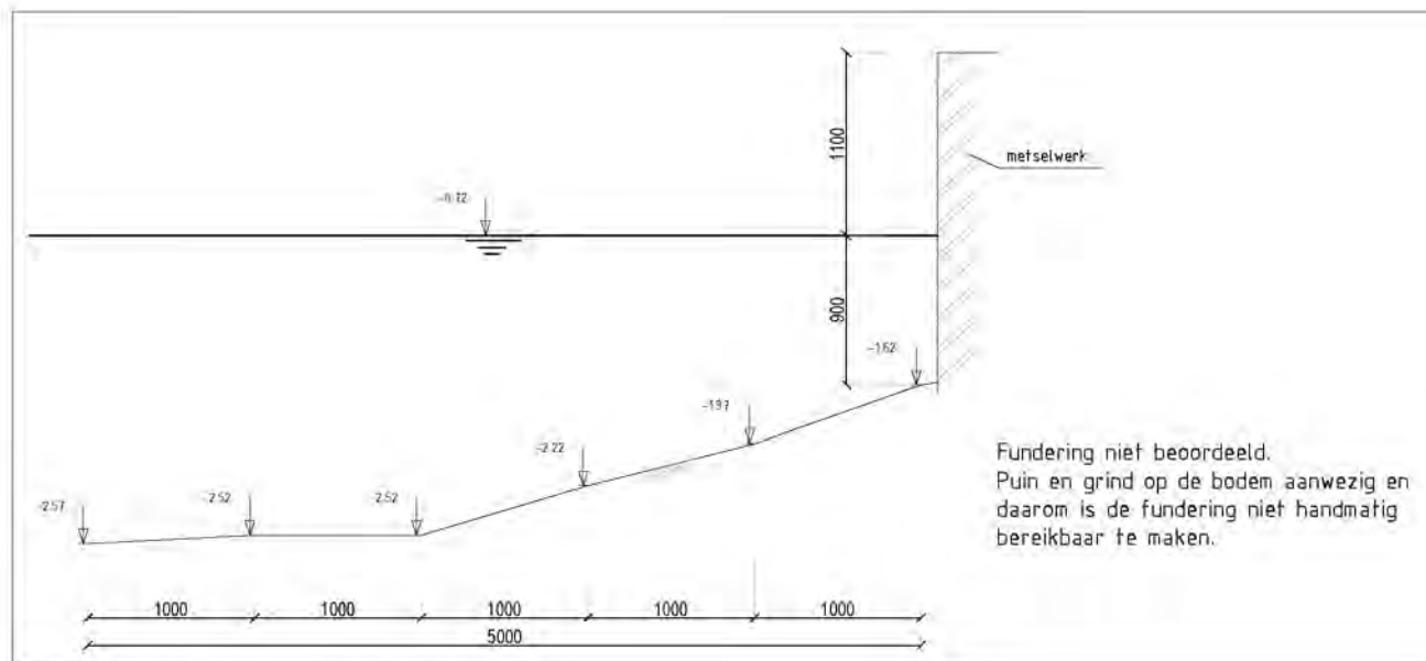
DOORSNEDE CONSTRUCTIE 001006a L-IP11 SCHAAL 1:50
