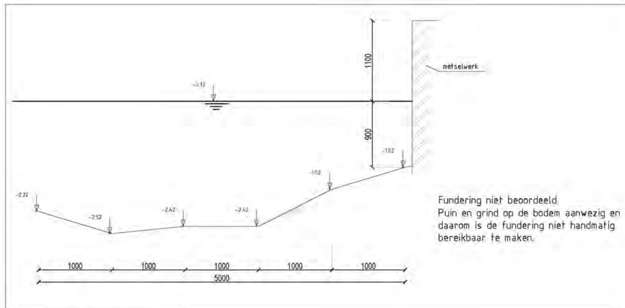
DOORSNEDE CONSTRUCTIE 001006a L-IP12 SCHAAL 1:50
