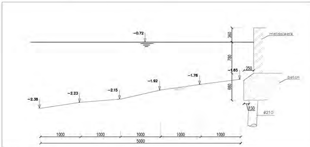
DOORSNEDE CONSTRUCTIE 001009a L-IP3 SCHAAL 1:50
