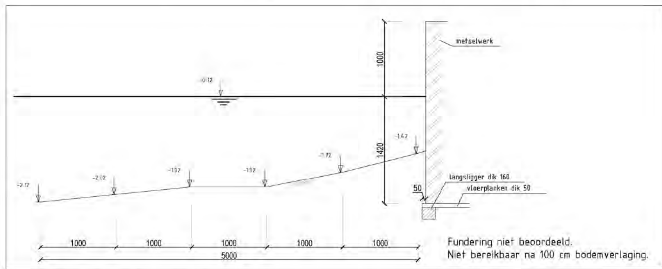
DOORSNEDE CONSTRUCTIE 001008 DEEL 1 L-IP14 SCHAAL 1:50
