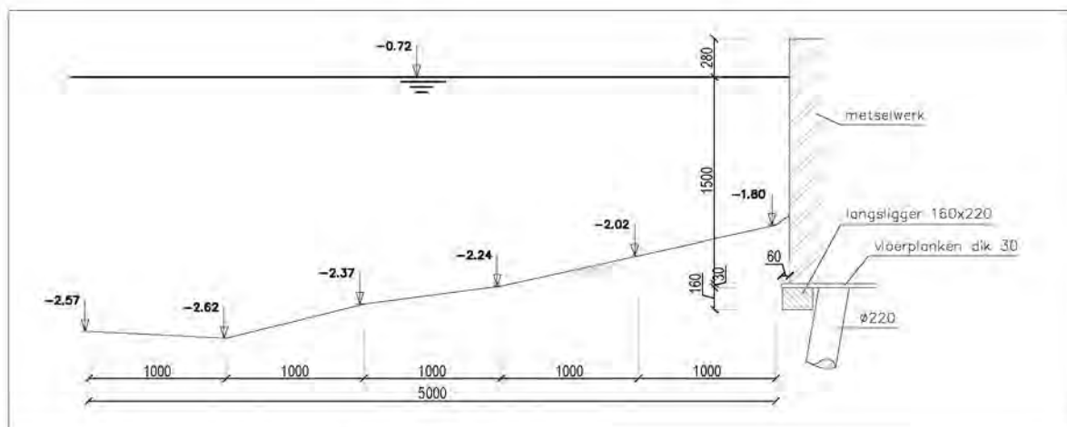
DOORSNEDE CONSTRUCTIE 001009 DEEL 2 L-IP2 SCHAAL 1:50
