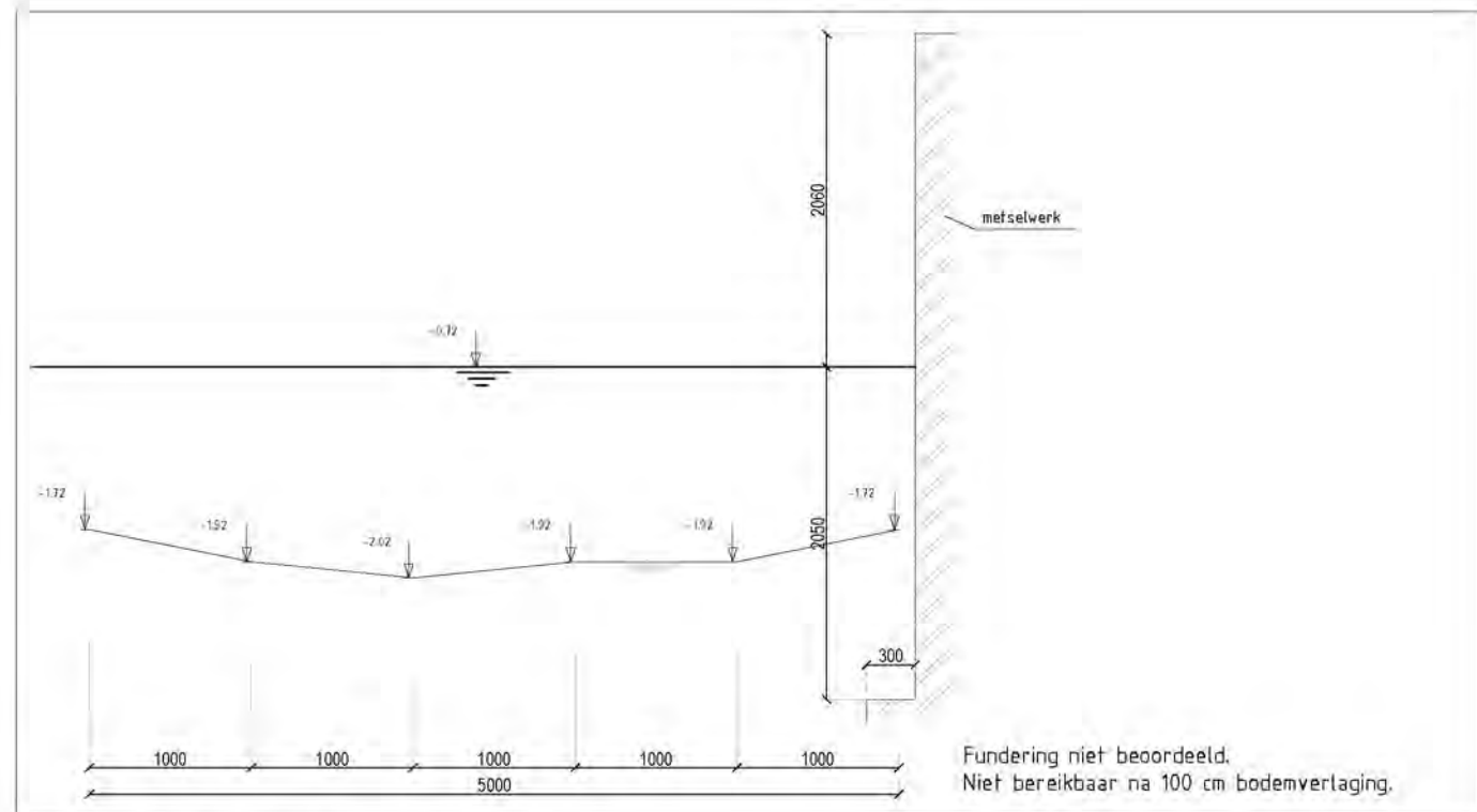
DOORSNEDE CONSTRUCTIE 001008 DEEL 2 L-IP16 SCHAAL 1:50
