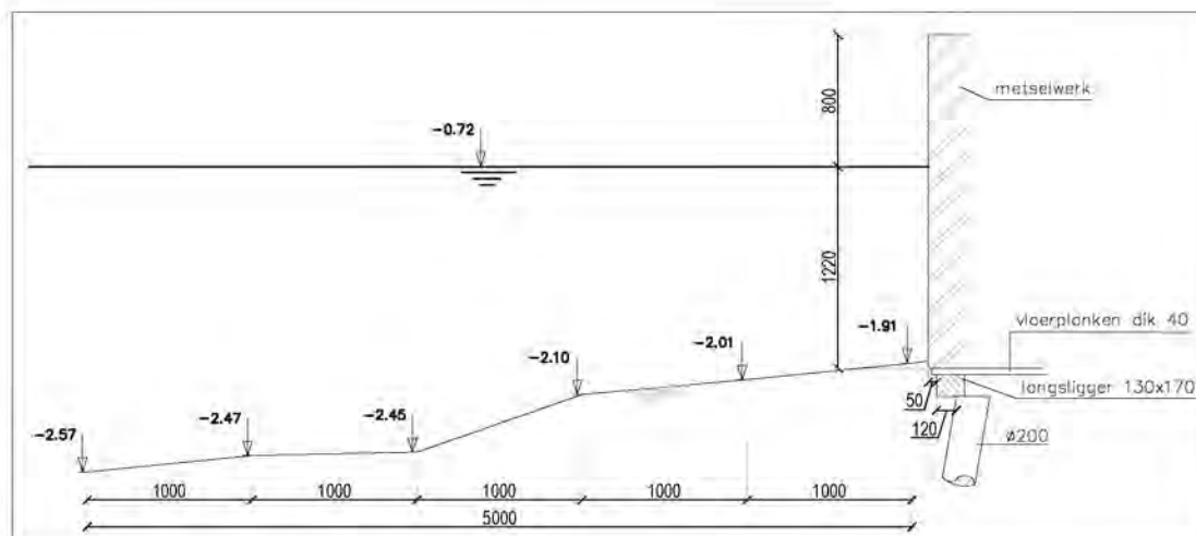
DOORSNEDE CONSTRUCTIE 001006 DEEL 1 L-IP5 SCHAAL 1: 50
