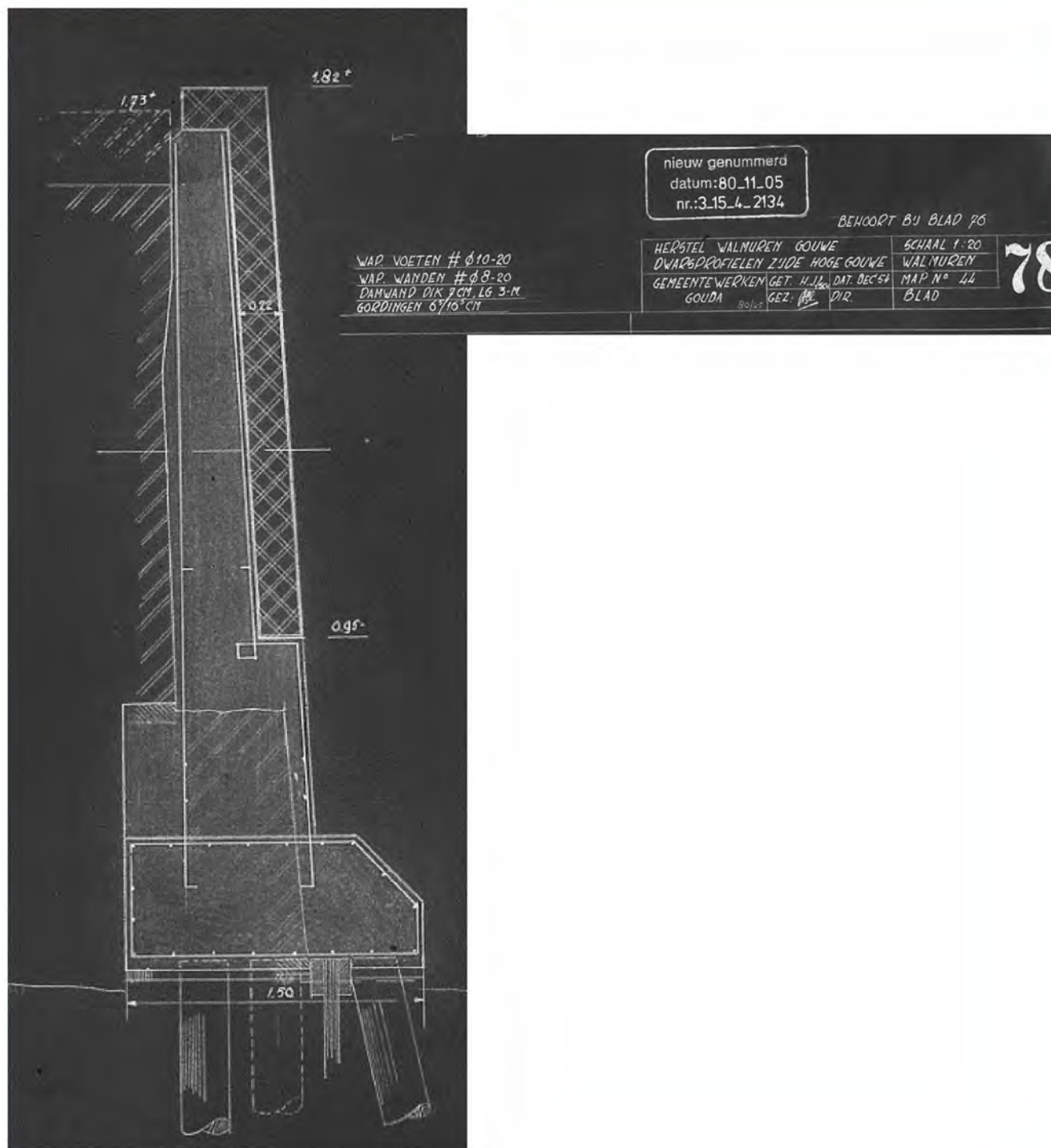
Foto 07: Dwarsdoorsnede van de walmuur
