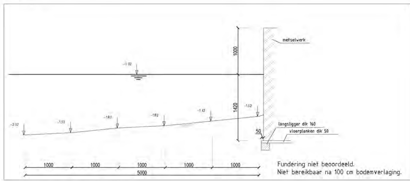
DOORSNEDE CONSTRUCTIE 001008 DEEL 1 L-IP15 SCHAAL 1:50
