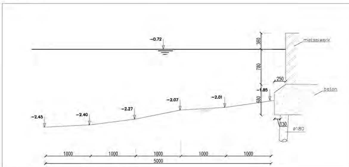
DOORSNEDE CONSTRUCTIE 001009a L-IP4 SCHAAL 1:50
