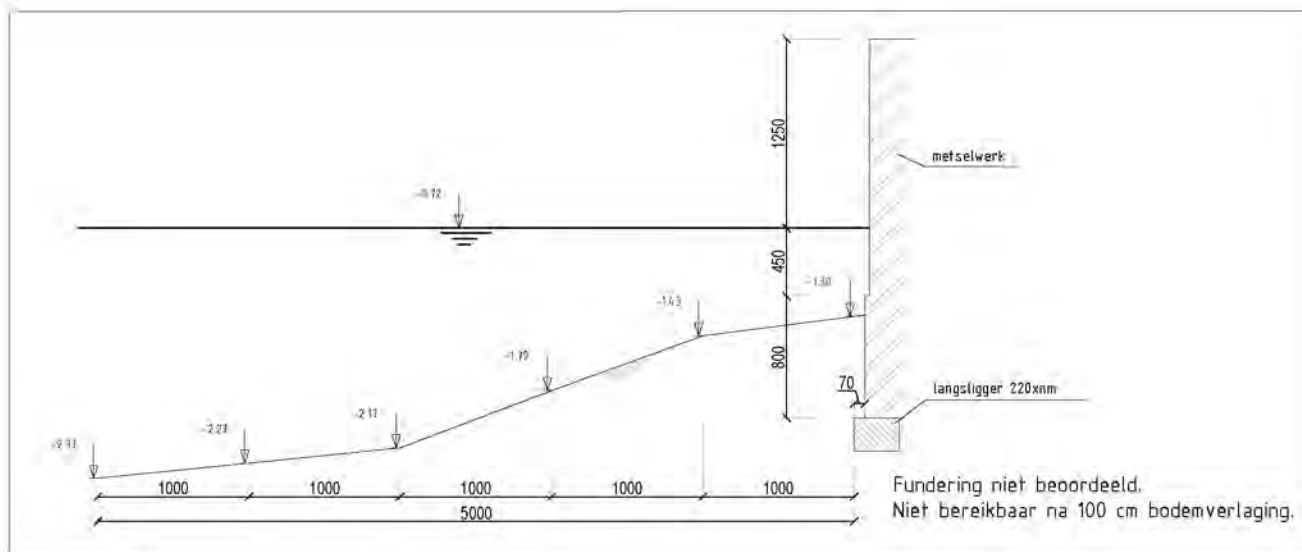
DOORSNEDE CONSTRUCTIE 001009 DEEL 1 L-IP1 SCHAAL 1:50
