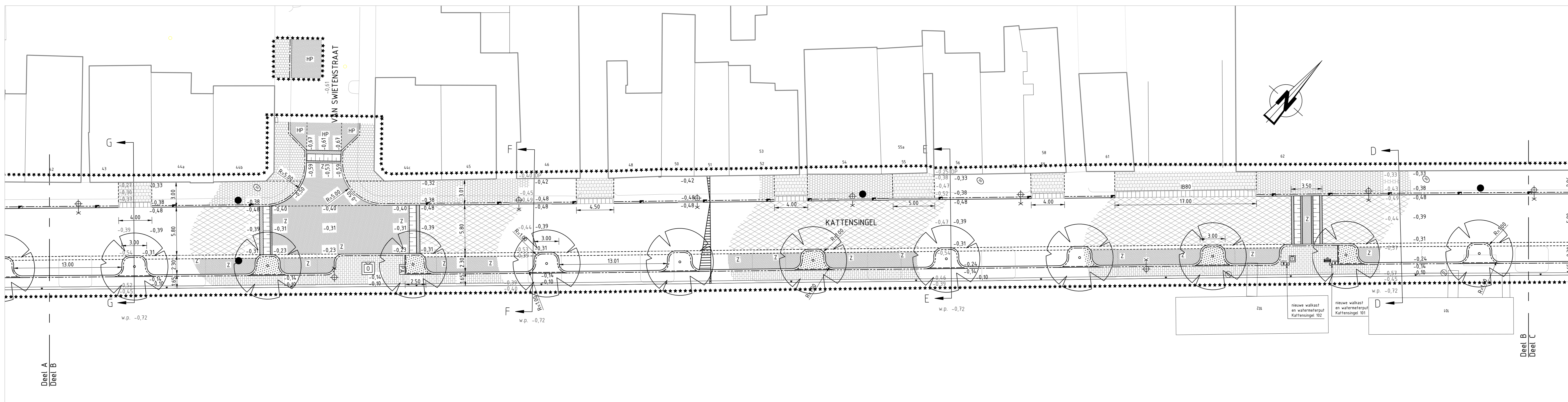
Kattensingel, Deel B SCHAAL 1:200
